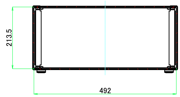
A-A (1:7.5)
